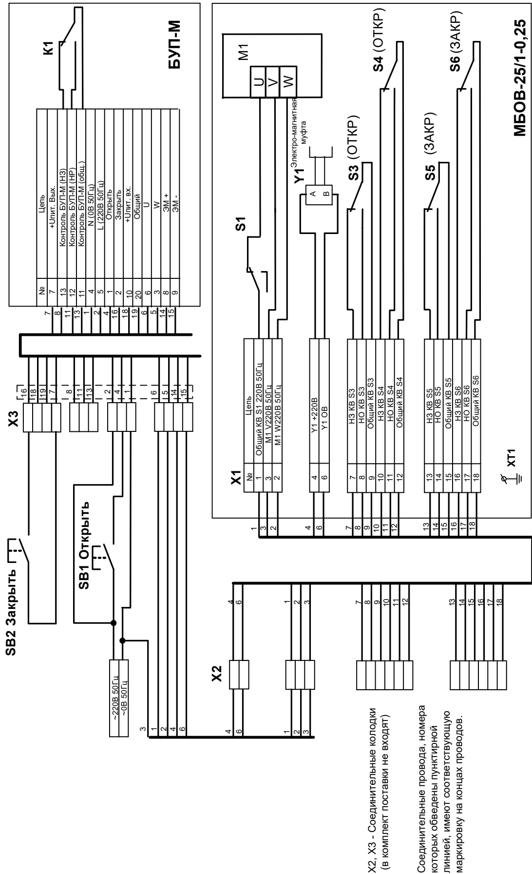
Схема электрических соединений БУП-М с электромеханизмом МБОВ-25/1-0,25 при отсутствии на объекте напряжения 220 В постоянного тока
